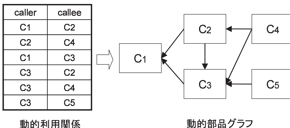
図 5.1: 支配部品グラフの例
