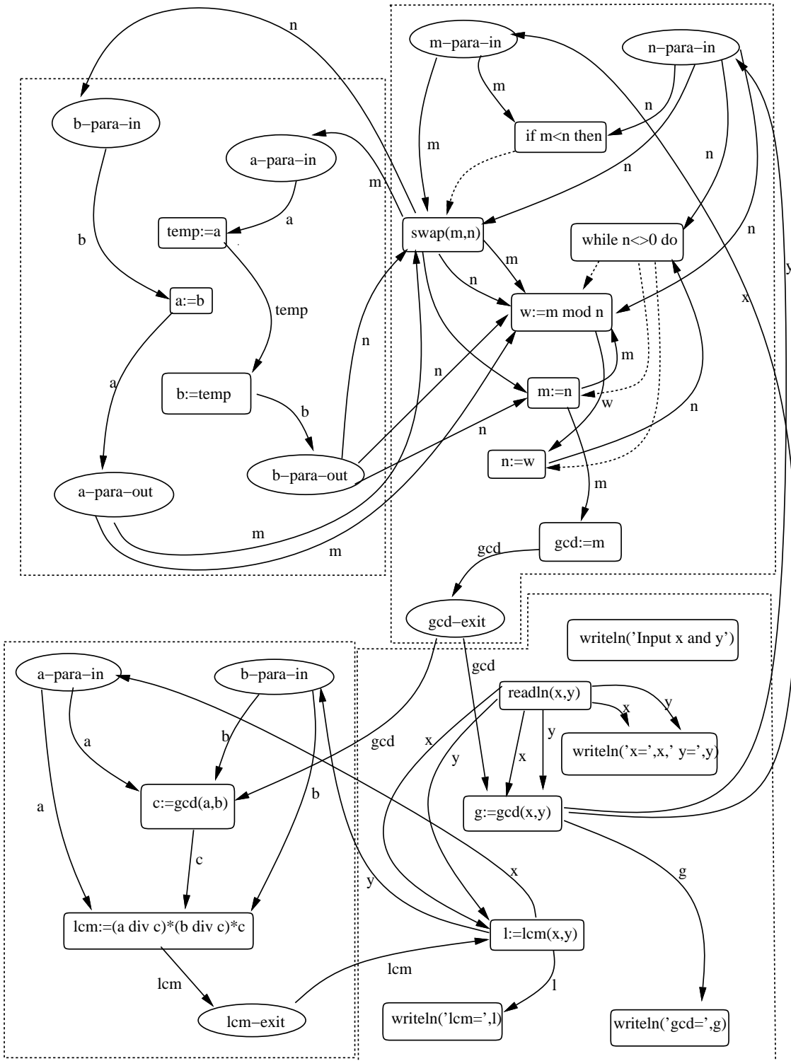
図2 PDGの例
