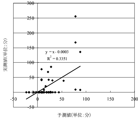
図 10 クラス分類を用いないエラー修正時間予測 (外れ値を除く) Fig. 10 Error fix time estimation except outliers without classi
