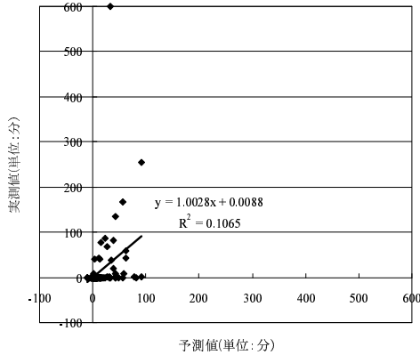
図 8 クラス分類を用いないエラー修正時間予測 (全データ) Fig. 8 Error fix time estimation by all data without classifi
