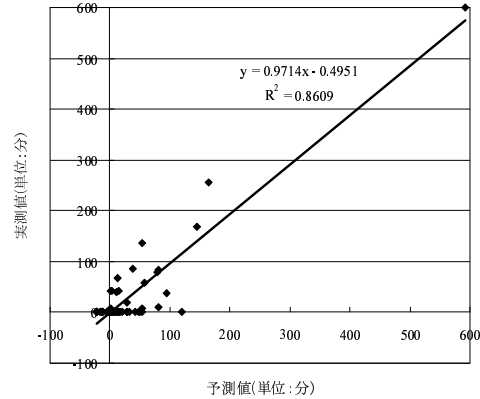
図 9 クラス分類を用いた修正時間予測 (全データ) Fig. 9 Error fix time estimation by all data with classification
