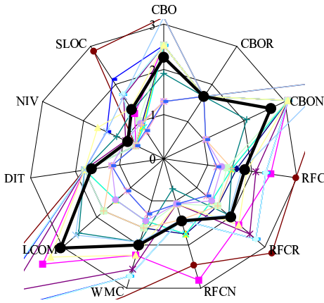
図 2 分類 CDialog のメトリクス値 Fig. 2 Metric values for CDialog classes
