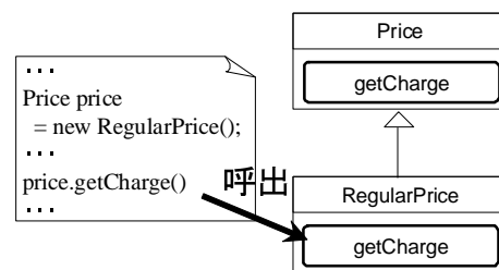
(b) ソースコード編集後
