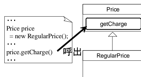
(a) ソースコード編集前
