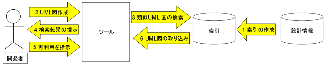
図 1 提案手法の概要
