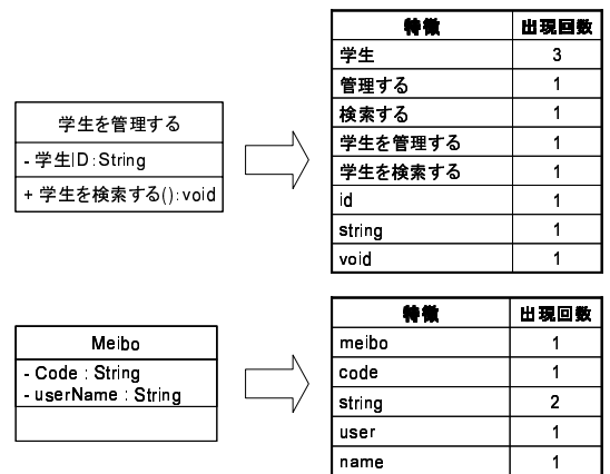
図 2 特徴の抽出例
