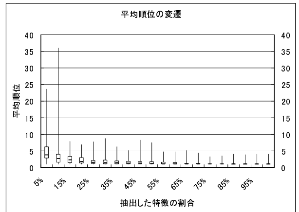
図 9 平均順位の変遷
