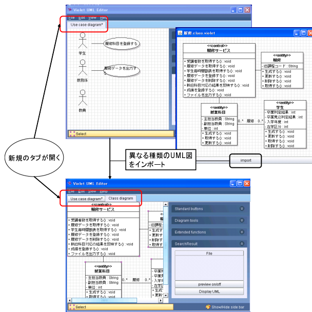
図 8 編集中の図と異なる種類の UML 図のインポートを行うと，新規のタブが開かれ，そこにインポートされる。
