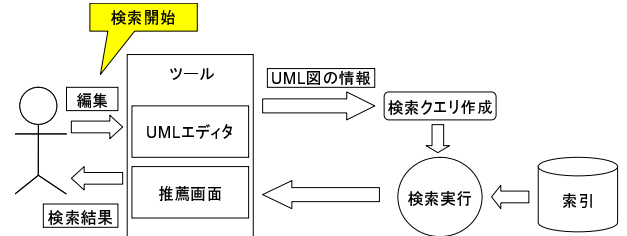
図 4 検索の流れ
